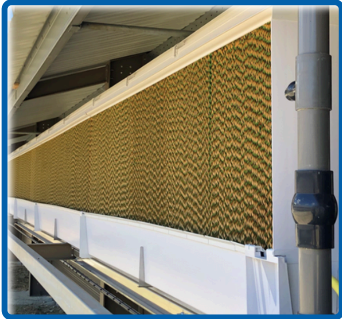
REFROIDISSEMENT PAR SYSTEME PAD COOLING
